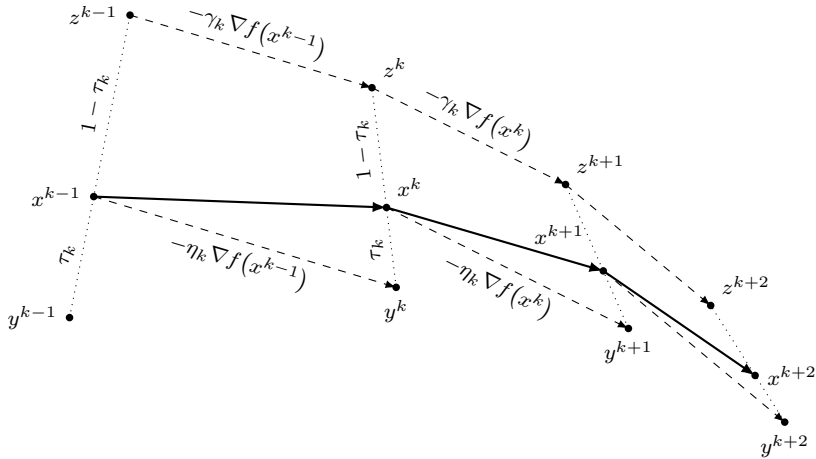
Рис. Л1.6: Три шага линейного каплинга. Пунктир — градиентные шаги для y и z вдоль градиента в точке x , сплошные линии — вычисление x^k как выпуклой комбинации.
