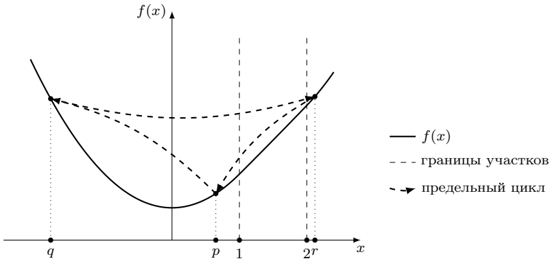
Рис. Л11.2: Иллюстрация предельного цикла в методе тяжёлого шарика на кусочно-гладкой функции f(x) .
