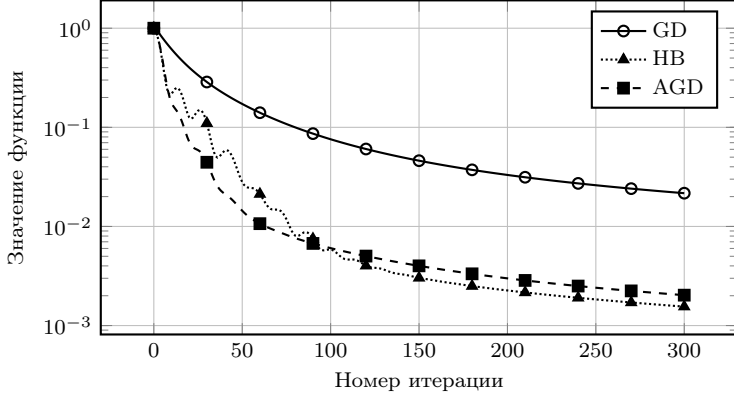
Рис. Л1.5: Сравнение методов GD (Алгоритм ??), Heavy Ball (Алгоритм Л1.1) и AGD (Алгоритм Л1.2) при неоптимальном подборе параметров на квадратичной задаче.
